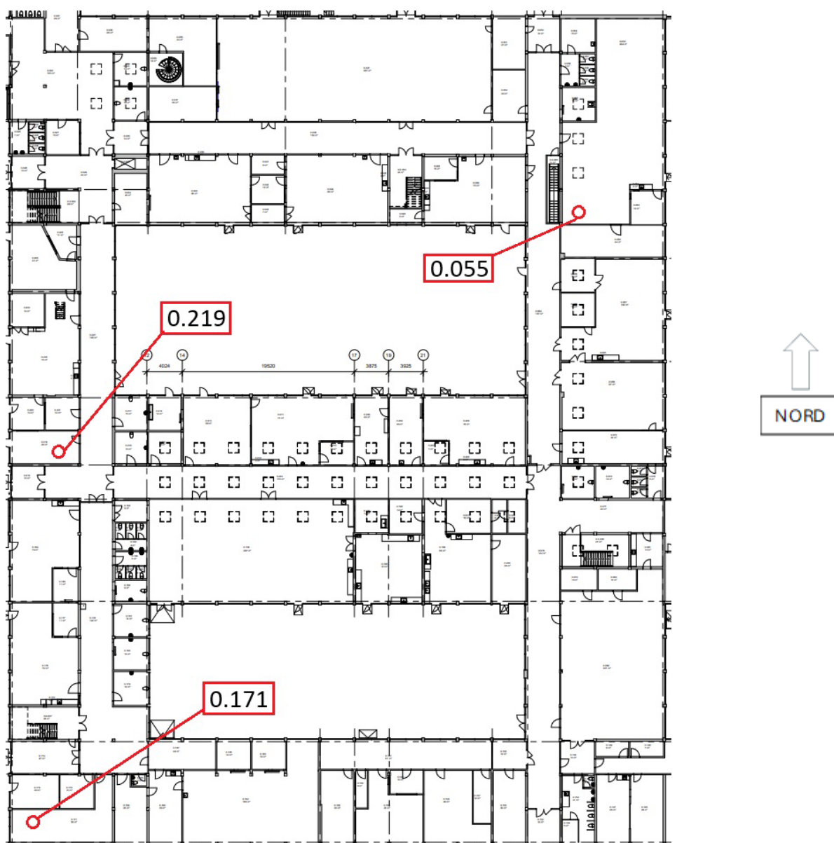
Figur 1. Plantegning for stuetagen i JAC med markering af prøvelokationer
