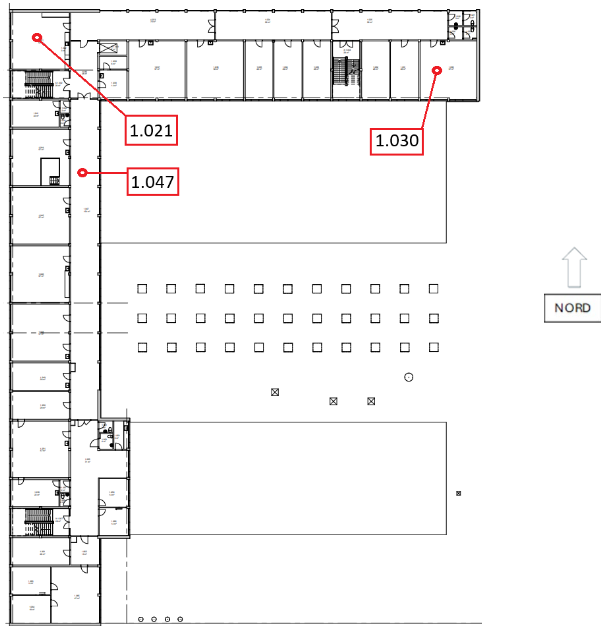
Figur 2. Plantegning for 1. sal i JAC med markering af prøvelokationer
