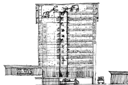
Nedrivning ved klipning med små maskiner inde i bygningen – mindre stykker beton føres igennem elevatorskakt og køres væk.
